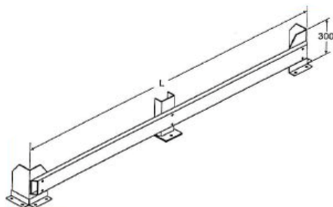
Sabot standard de longueur 1200 ou 2500 mm Section de la protection : 120 x 40 mm
